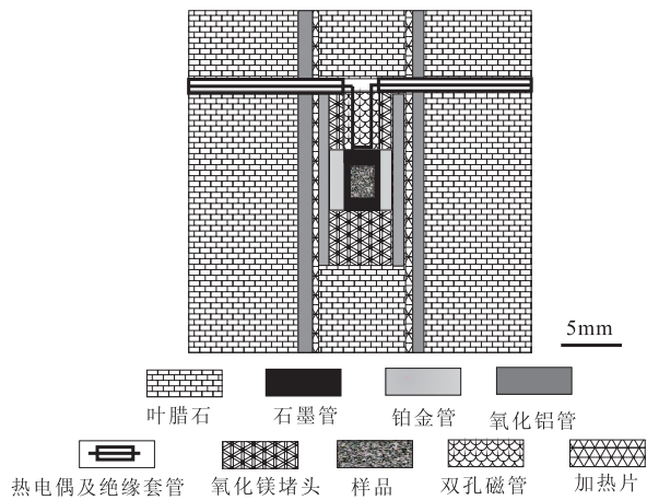
图 2 实验样品组装示意图
