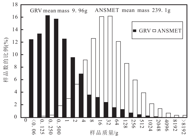
图3 格罗夫山陨石质量分布特征(据文献[13])
