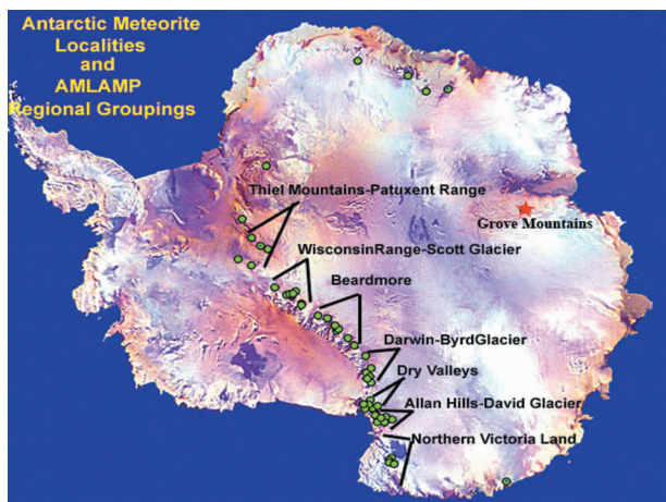
图 1 南极陨石富集区的分布图(据文献[4]修改)
