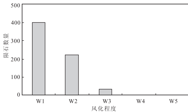
图5 格罗夫山陨石风化程度统计(据文献[30])
