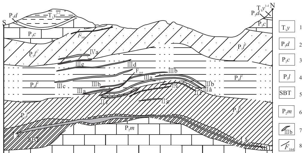
1-夜郎组;2-大隆组;3-长兴组;4-龙潭组;5-构造蚀变体;6-茅口组;7-矿体及编号;8-断层及编号
