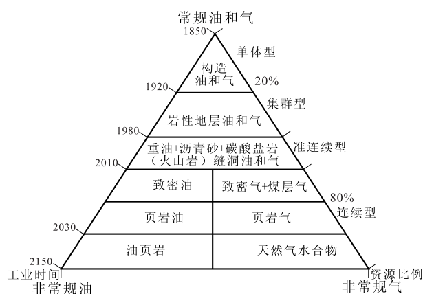
图1 油气资源类型特征三角图
