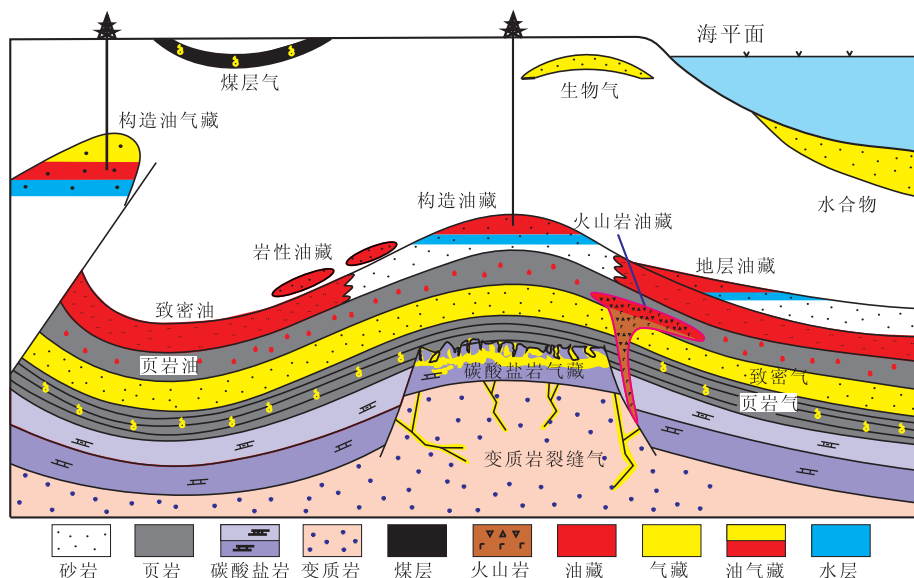
图3 常规与非常规油气聚集类型分布
