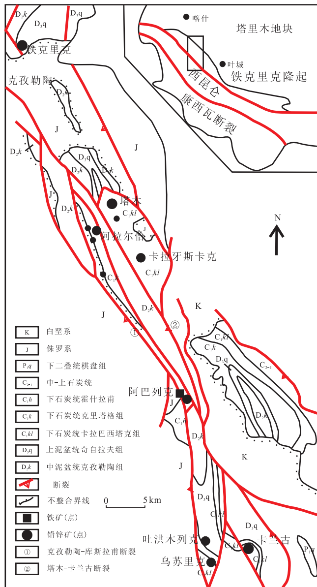
图 1 塔西南缘铅锌矿带地质矿产简图
